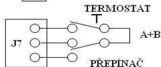
Obr.6 – příklady zapojení dálkového ovládání/hodin
