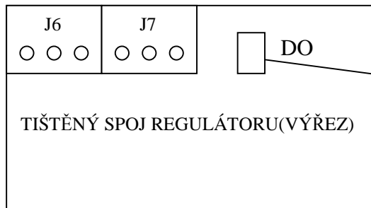
Obr.3 - připojení dálkového ovládání do svorek J7
