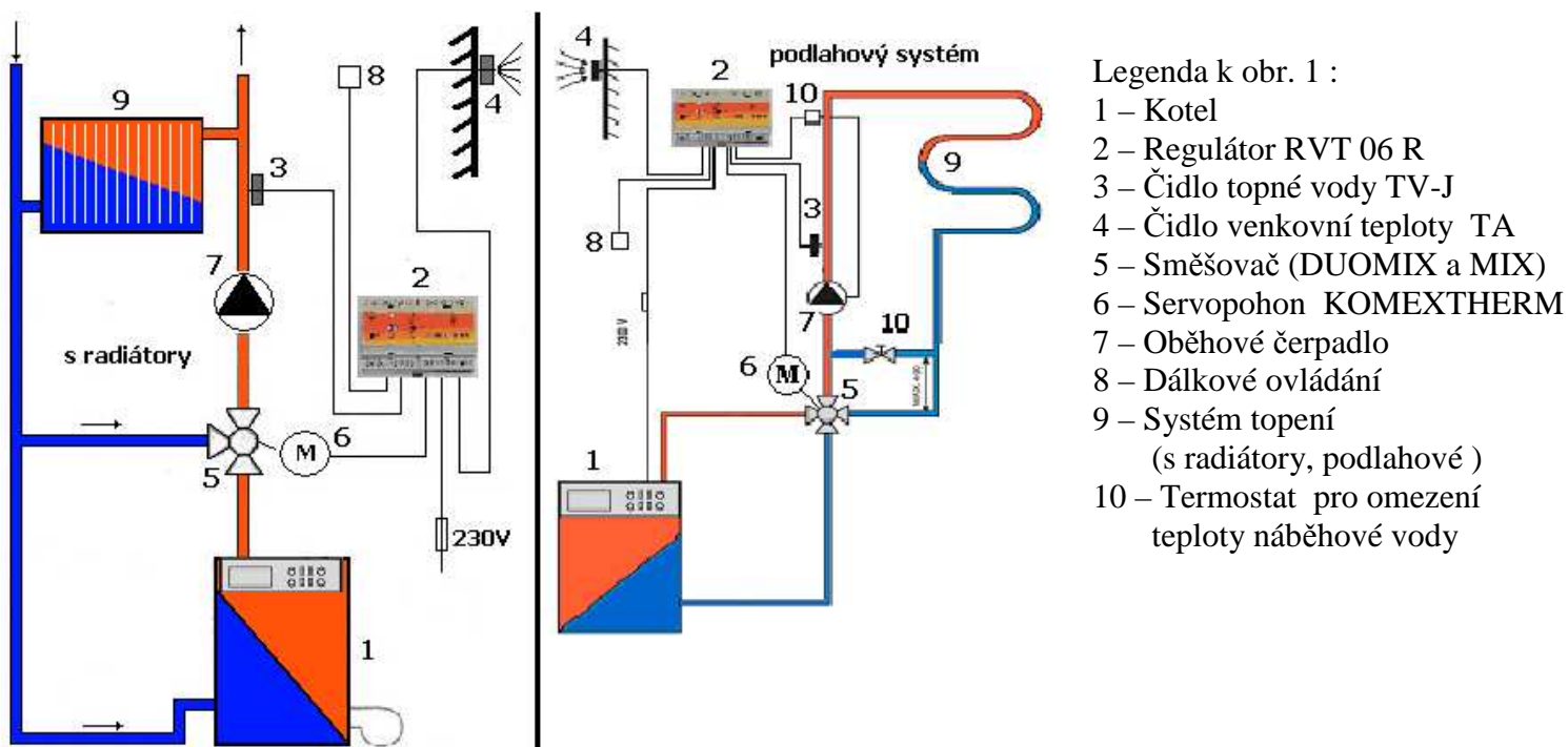
Obr. 1 – příklady topných systémů řízených regulátorem RVT 06 R se směšovači DUOMIX a MIX ( s radiátory a podlahové systémy )
