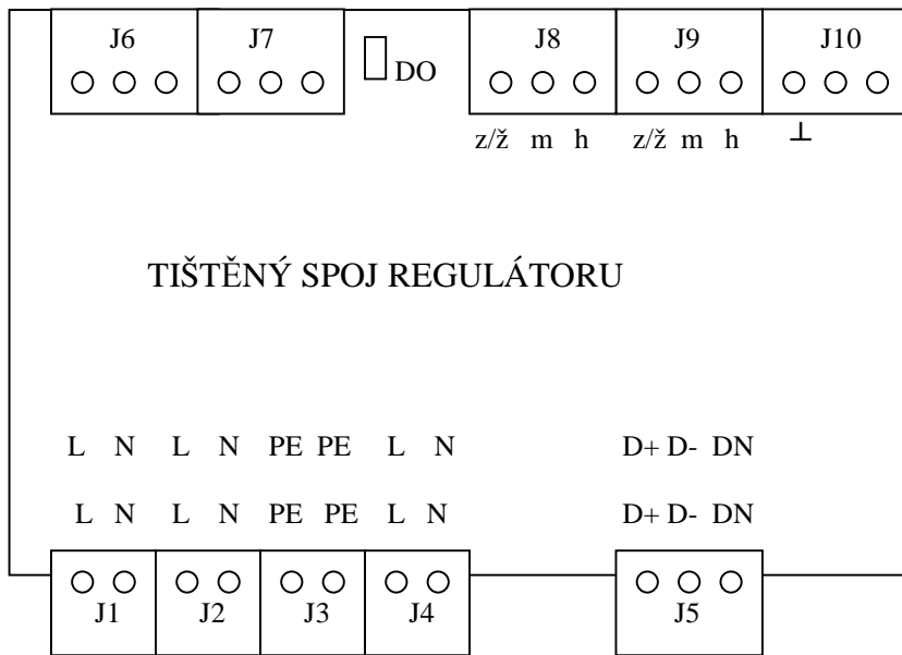
Obr.2- Svorkové schéma regulátoru RVT 06 R
